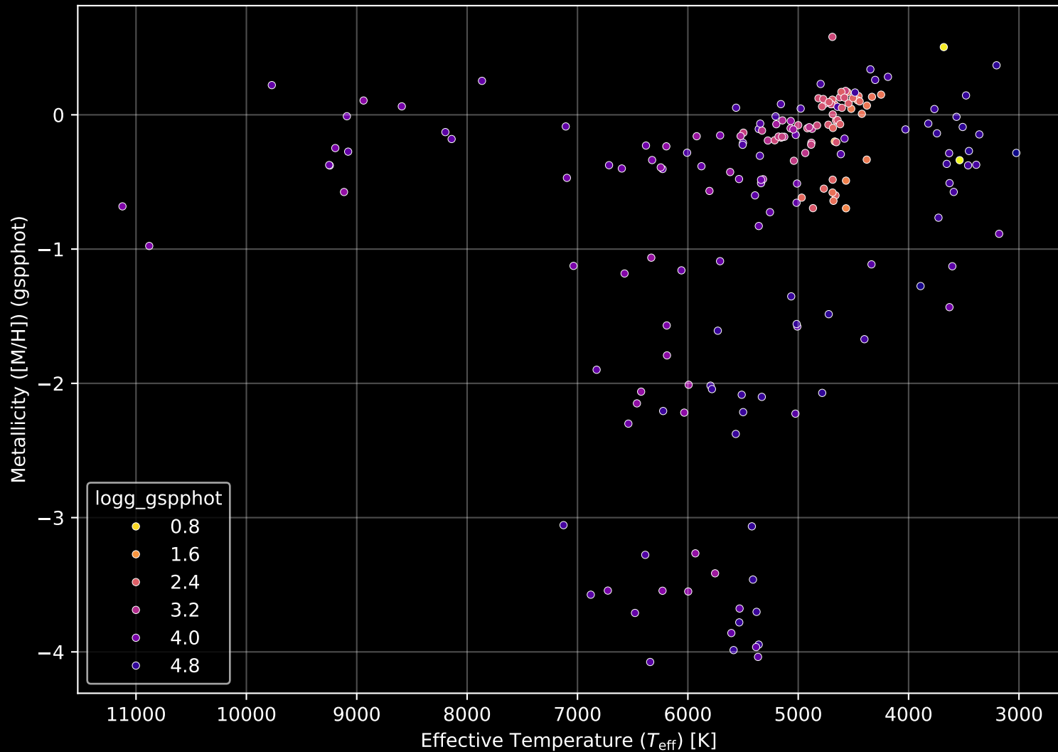
APOGEE DR17 Field: [K2_C7_008-12_bt] Stellar Population Parameters (n= 196)
